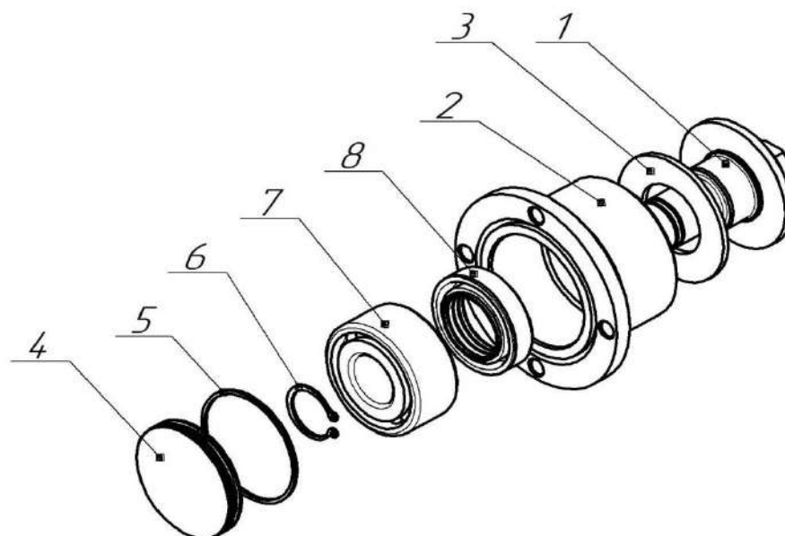
КДК-4.60.200 Ступица
