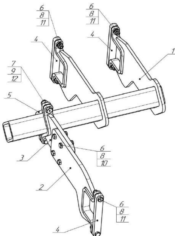
АДК-4.00.650 Стяжка
