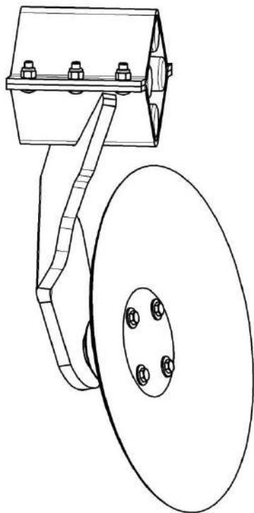
АДК-4.04.000 Стойка дисковая.
