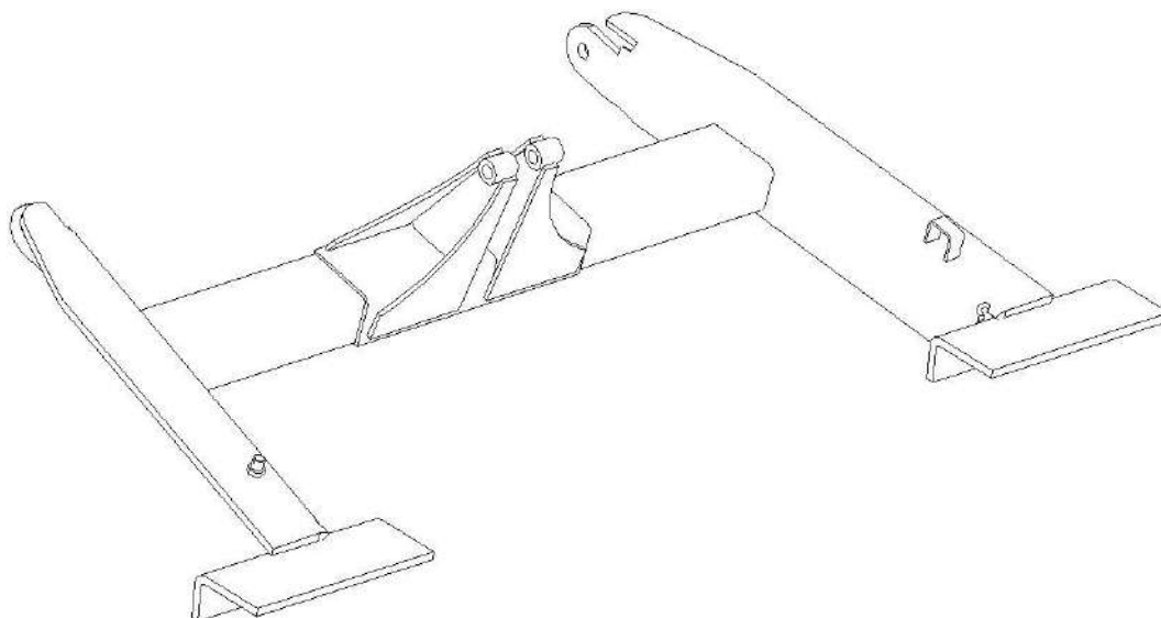
КДК-4.08.000 Кронштейн
